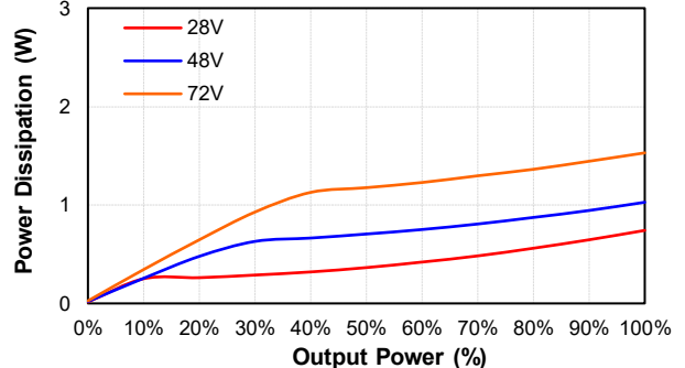
NCS01W8-48S240 Pd Vs Po @25 Deg. C
